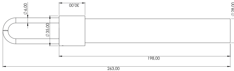
SS-43HTC2 Yüksek Sıcaklık Korumalı Şut Seviye Sensörü
